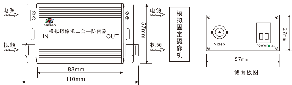
模拟摄像机二合一防雷器尺寸及接线图示
